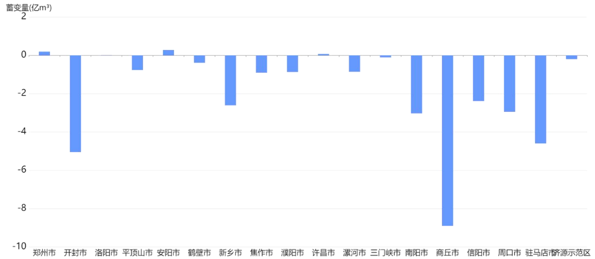
图 8 与上年同期相比河南省平原区浅层地下水蓄变量
