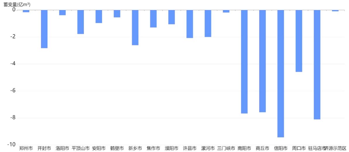
图 7 与上月同期相比河南省平原区浅层地下水蓄变量
